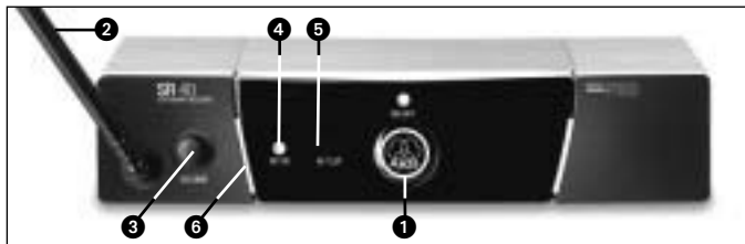
Fig. 1: Commandes de la face avant du récepteur
