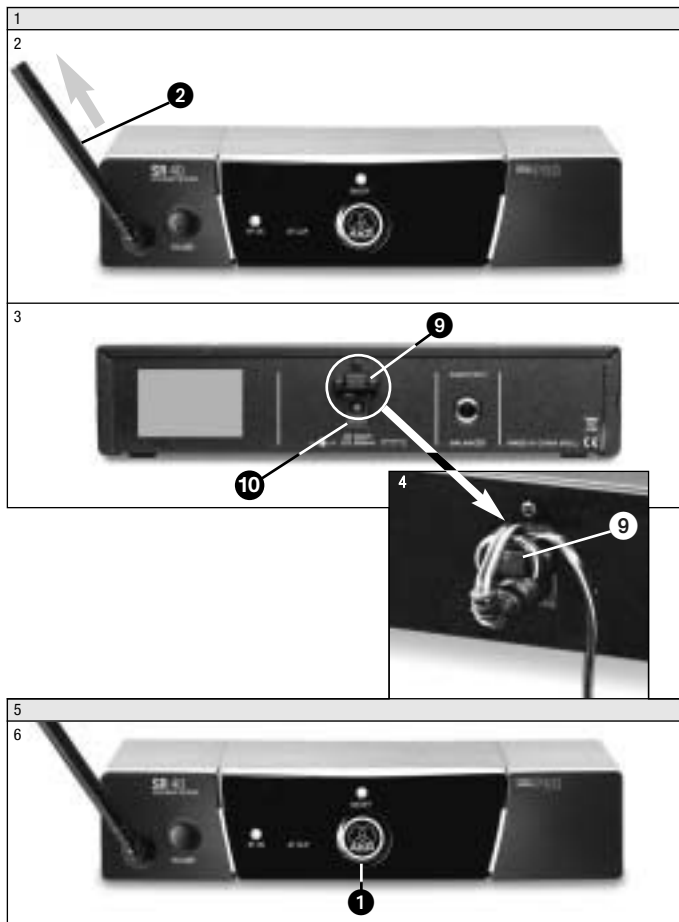
Fig. 5: Conexão à rede elétrica
