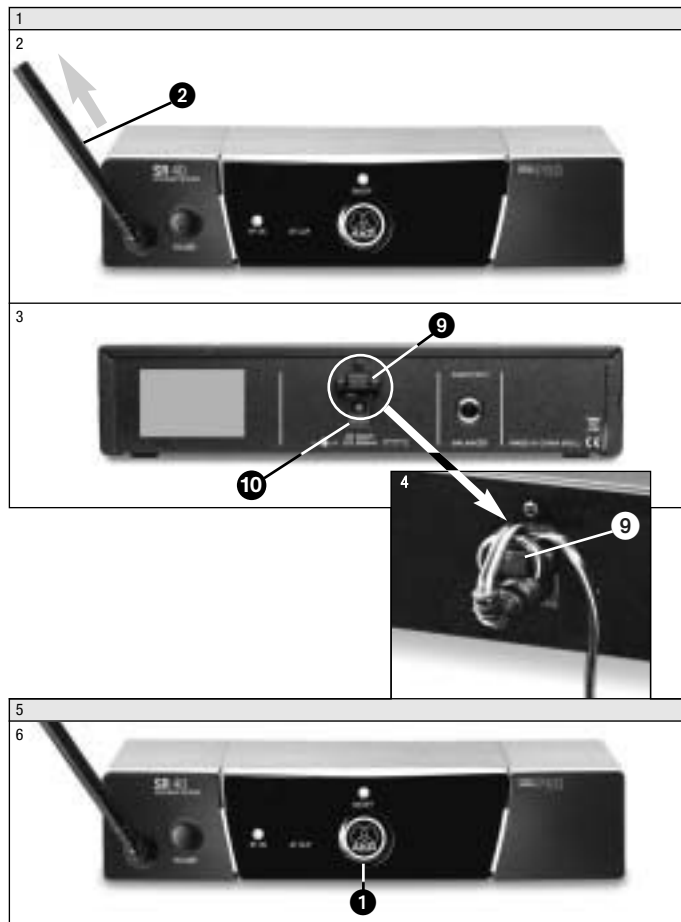
Fig. 5 : connexion au secteur
